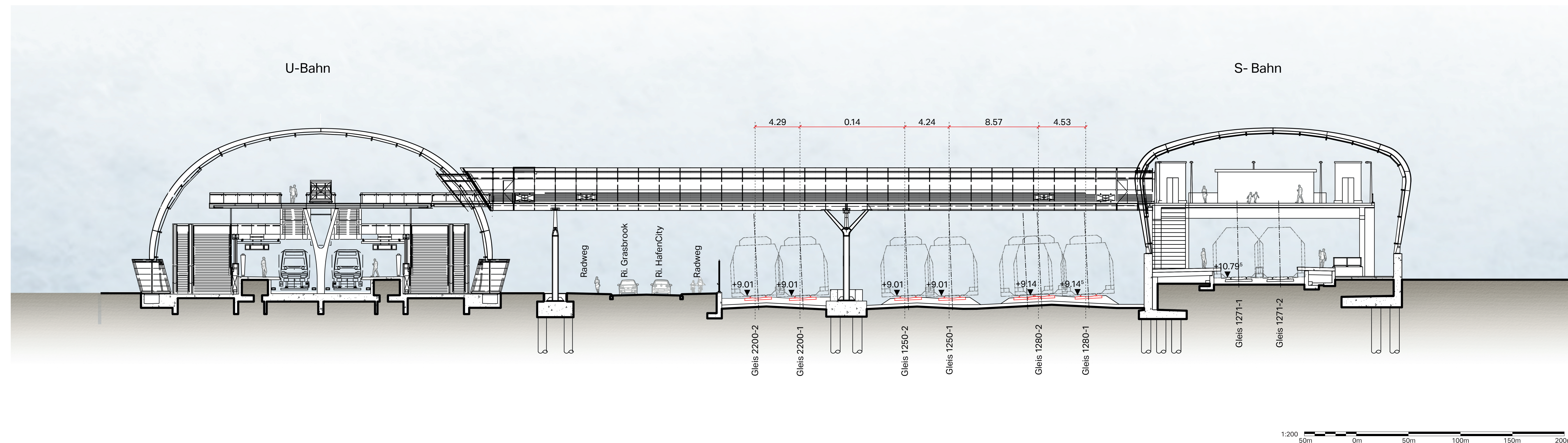
Schnitt C-C - Skywalk M 1:200
