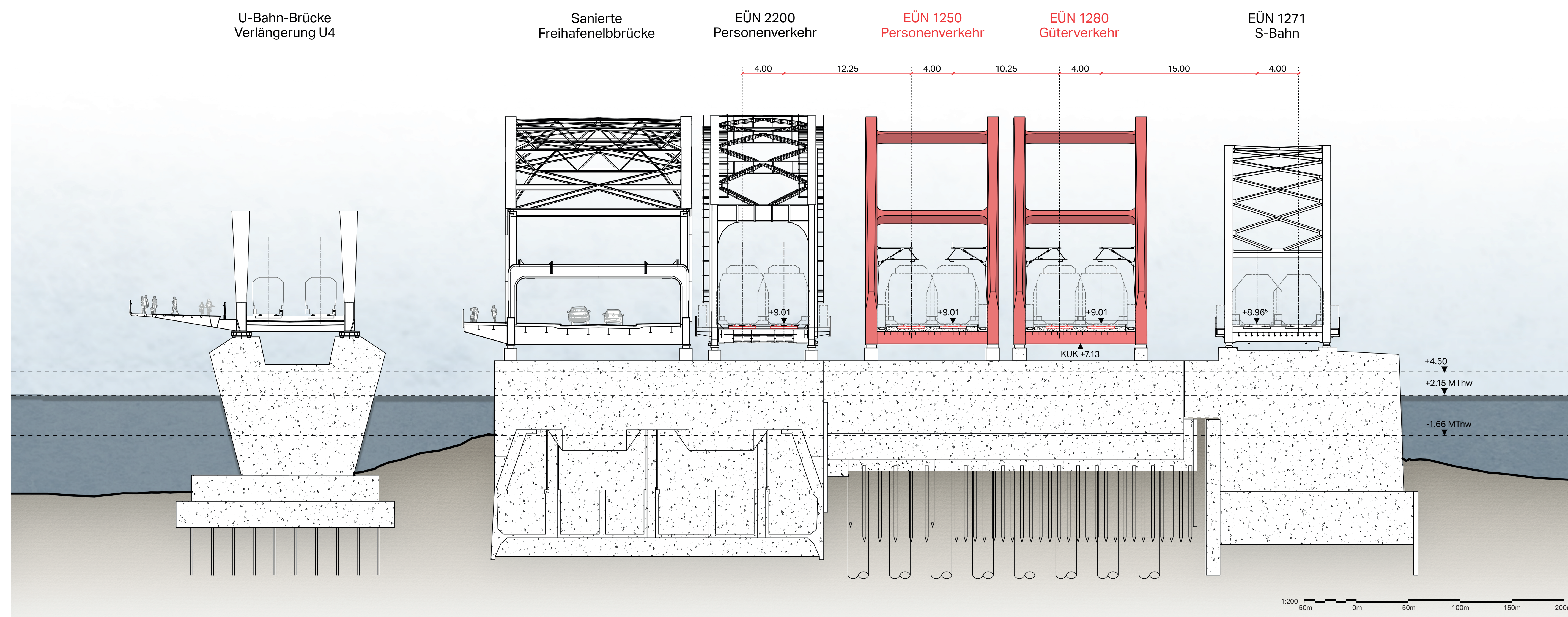
Schnitt B-B - Strompfeiler Nord M 1:200
