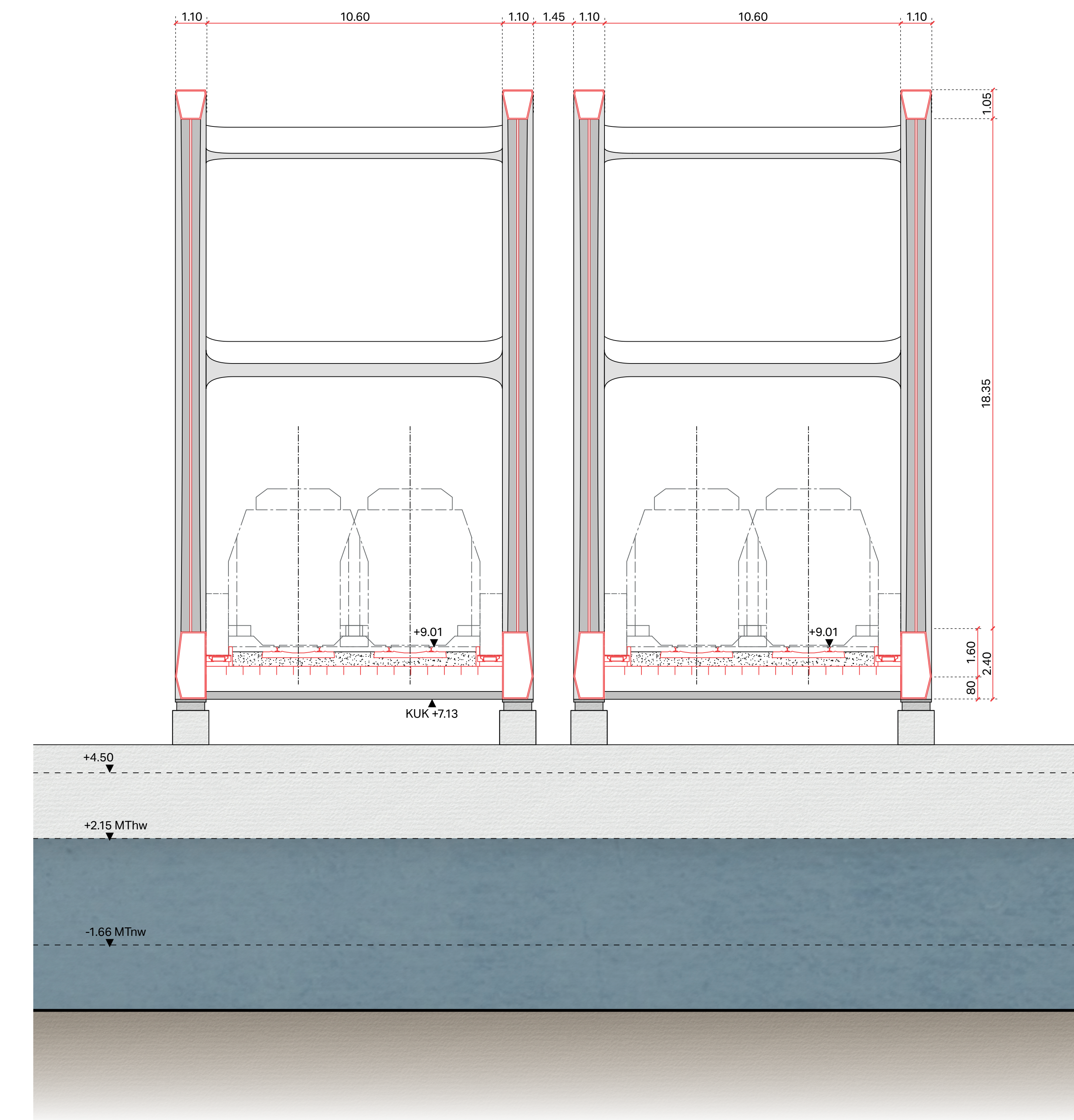
Querschnitt Feldmitte M 1:100
