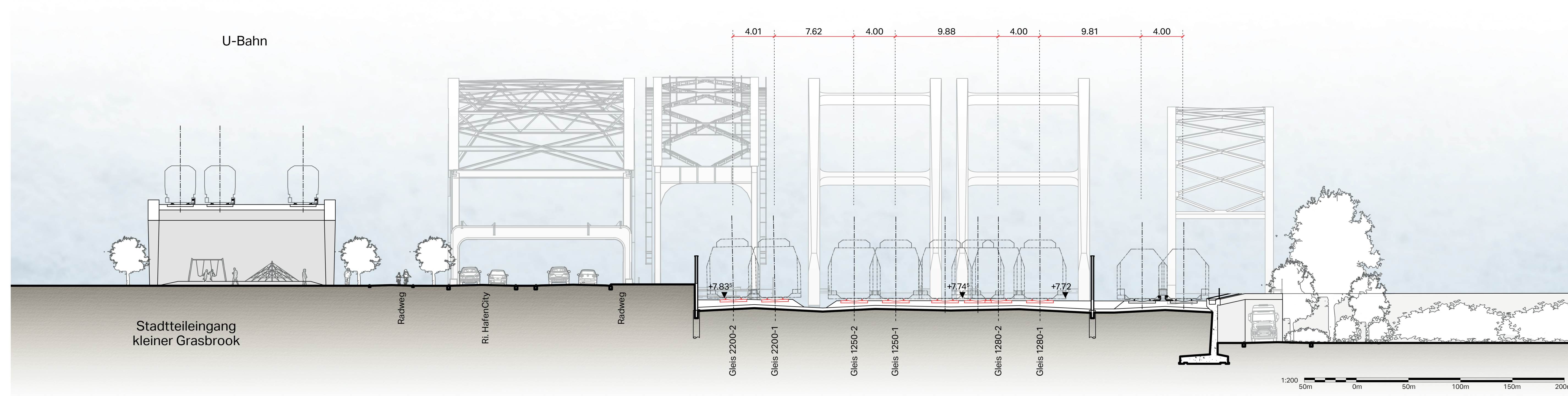
Schnitt A-A - Stadtteileneingang kleiner Grasbrook M 1:200
